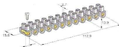
SORACO CXJU-30110
