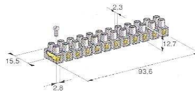
SORACO CXJU-30100
