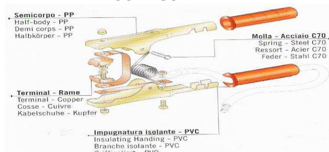
Alicate isolado vermelho 600 amperes
