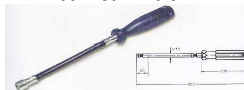
SORACO ABAS-CB7
