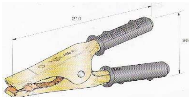
Alicate isolado preto 400 amperes
