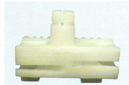
Kit reparação elevador Citroen Xsara Picasso Esquerdo
