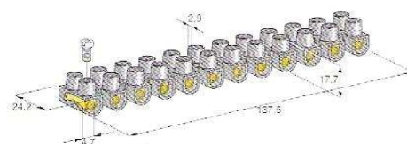
SORACO CXJU-30120
